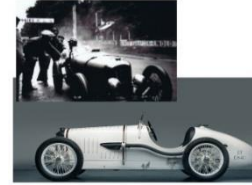
AMILCAR C6 COURSE 1100cc - 1928 - CHINE - N° 042
